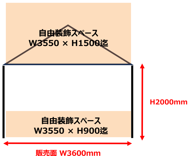
【立面図】
