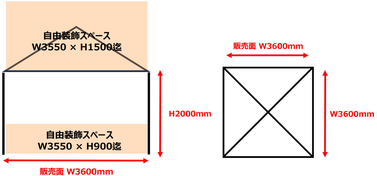
【立面図】
